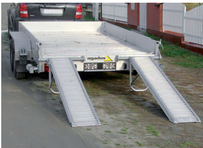
Hliníkový přepravník bagrů
