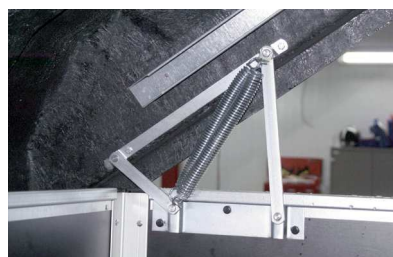
Jednoduchý systém uchycení a sklápění víka
